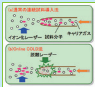
オンライン濃縮レーザー脱離試料導入法(Online COLD法)
